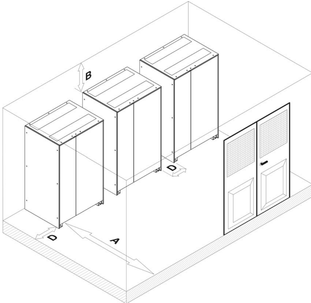
Illustration 5 – Dégagement minimum
